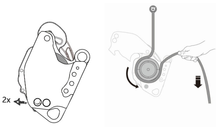
Рис 2 - Как заправить канат
