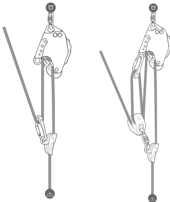
Рис 9 - Резервные системы
